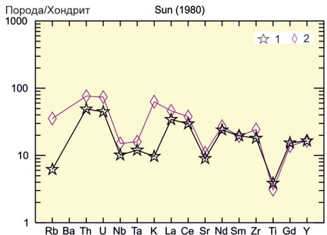
Рис. 5. Распределение мультиэлементных спектров в породах плагиогранитового комплекса, нормированных на хондрит [14]. Усл. обозн. см. на рис. 4
