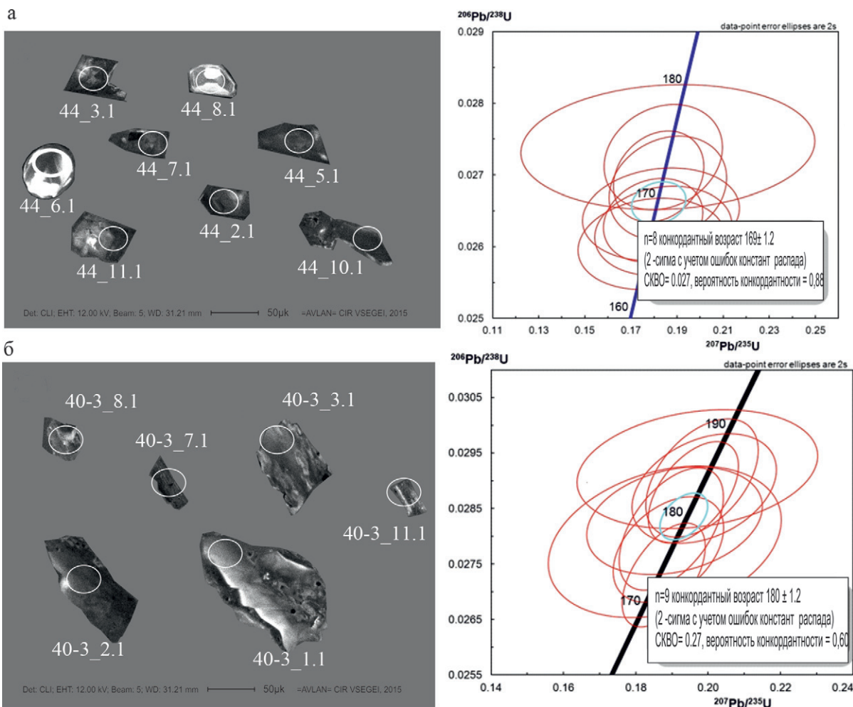
Рис. 7. Катодолуминесцентные изображения цирконов из плагิโอгранитового комплекса и построенные по ним конкордии
