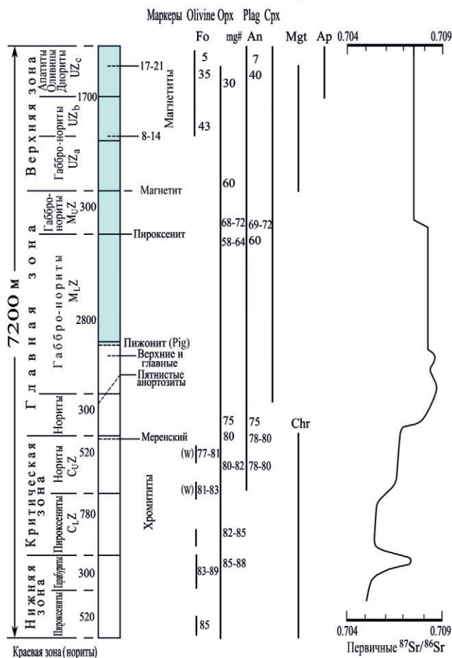
Рис. 2. Сводный вертикальный геологический разрез интрузивов Дюфек и Бушвелд
