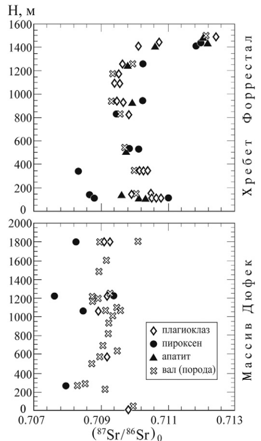
Рис. 8. Вариации первичных отношений ^{87}\text{Sr}/^{86}\text{Sr} в плагиоклазе, пироксене и вмещающих породах в зависимости от положения в разрезе горного массива Дюфек и хр. Форрестал
