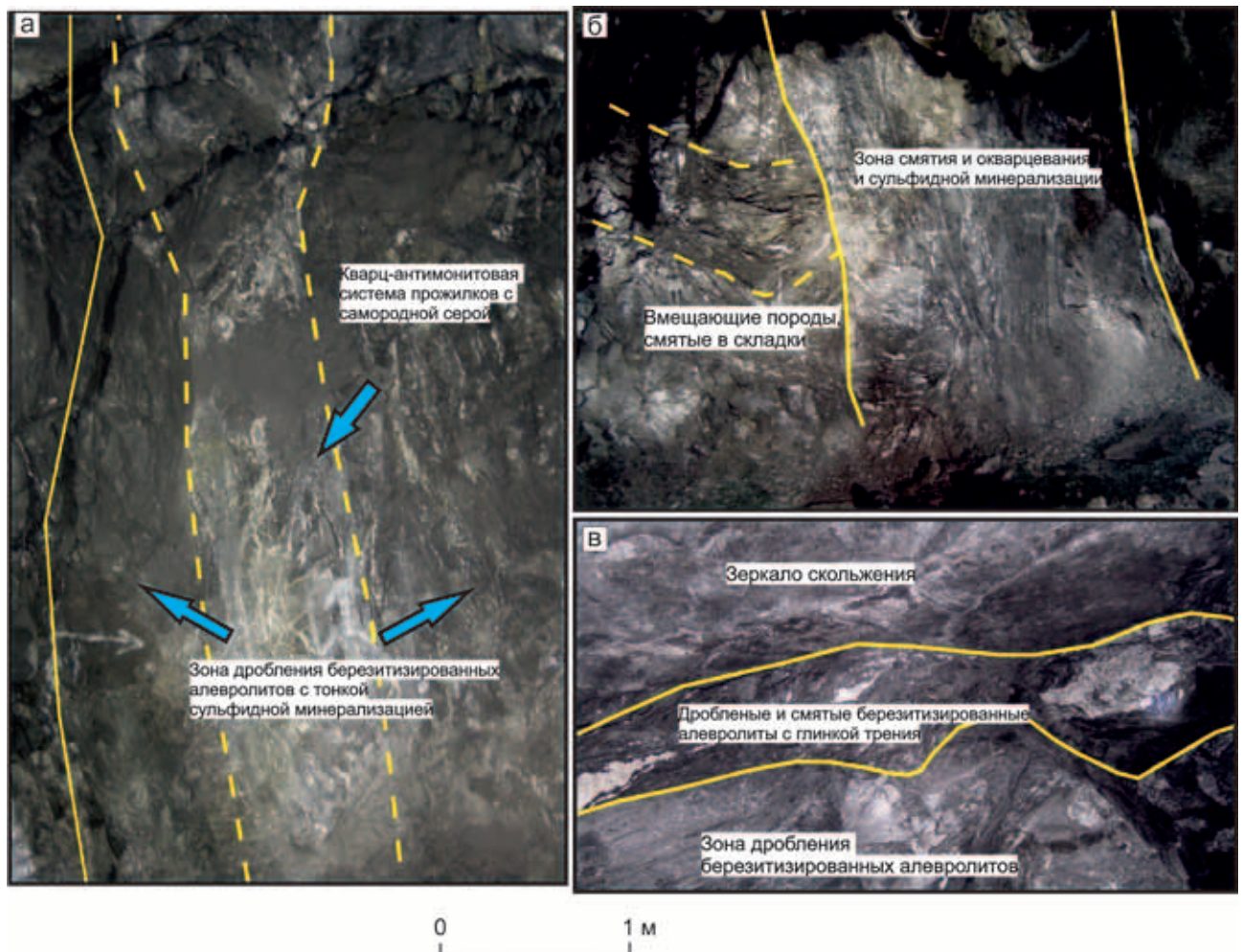
Рис. 4. Рудное тело № 1 в подземных горных выработках и его основные структурные элементы (фото автора) a и б – забой рудного тела (горизонты +80 и +100); в – кровля, горизонт +140
