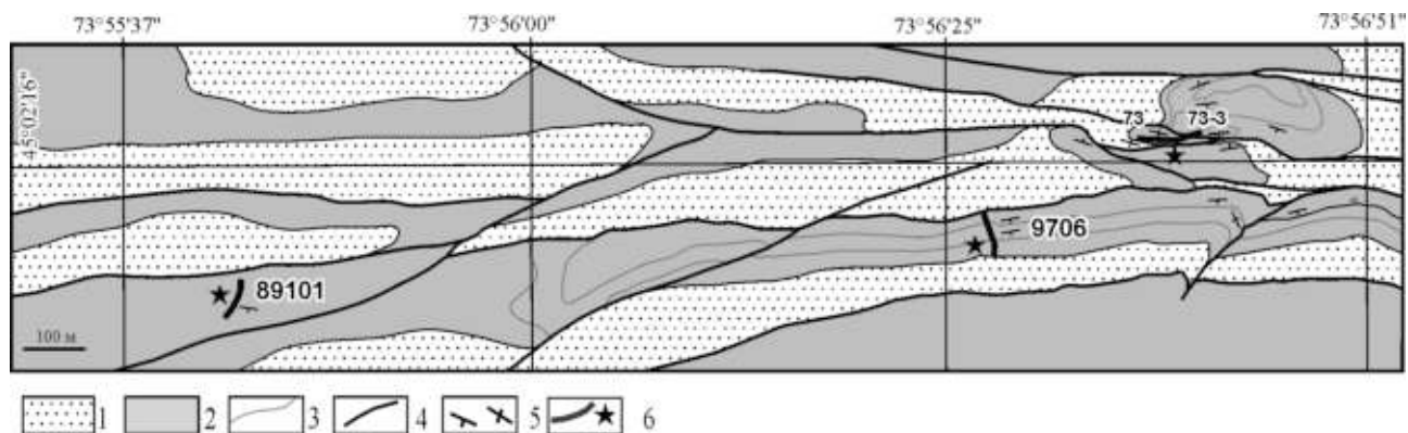
Рис. 5. Схема геологического строения участка разрезов Раковая гора (от т. н. 73 до т. н. 73-3) и Памятник природы (разрезы 89101 и 9706) (по данным А. В. Рязанцева, О. И. Никитиной и автора)
