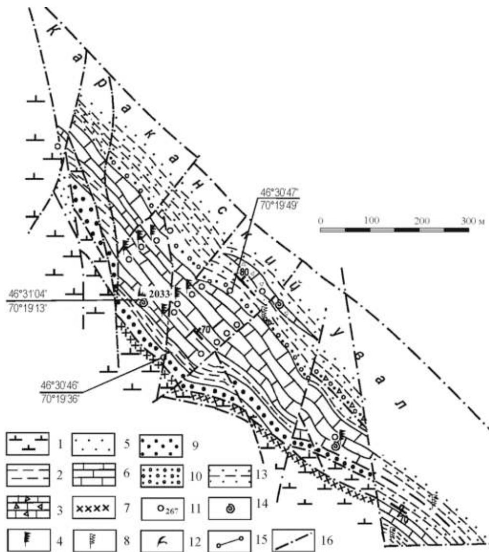
Рис. 32. Геологическая схема Караганского увала с указанием местонахождения отбора конодонтов, по [Никитину и др., 2008]
