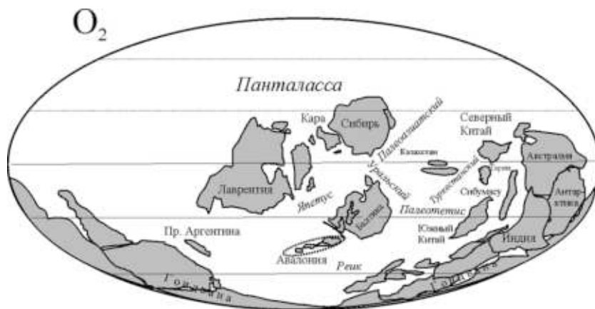
Рис. 40. Палеогеографическая реконструкция для среднего ордовика, по [Scotese, 2001; Cocks et Torsvik, 2002; Agematsu et al., 2006] с дополнениями
