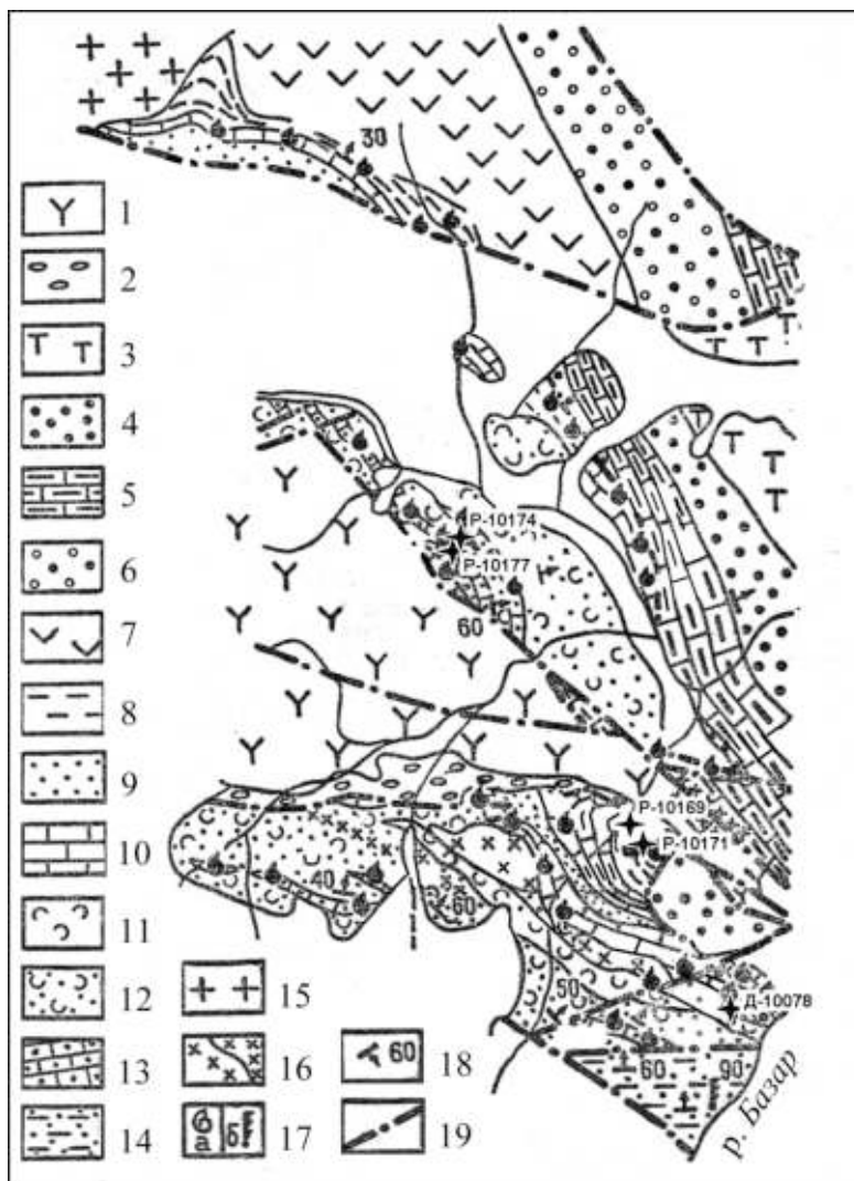
Рис. 26. Схема геологического строения правобережья р. Базар у выхода из хр. Тарбагатай, по [Никитин, 1972]
