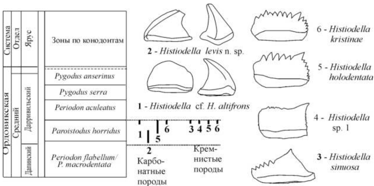
Рис. 71. Распространение видов рода Histiodella в карбонатных и кремнистых породах Казахстана. В кремнистой бурубайтальской свите все четыре вида Histiodella были найдены на одном стратиграфическом уровне
