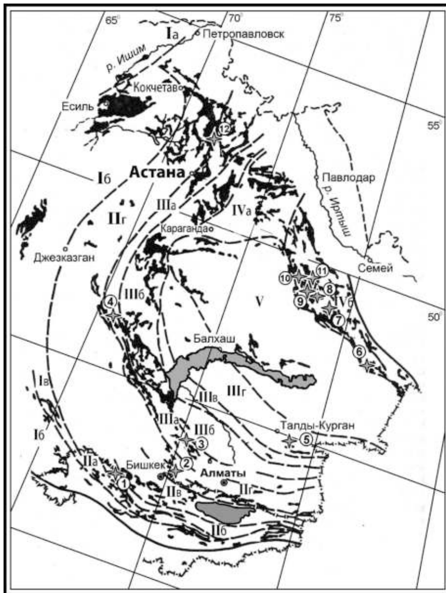
Рис. 17. Схема расположения изученных местонахождений конондотов в карбонатных отложениях Казахстана и Северной Киргизии (схема районирования ордовика палеозойд Казахстана и Киргизии, по [Решения ... , 1991] (структурно-тектонические зоны см. на рис. 1)
