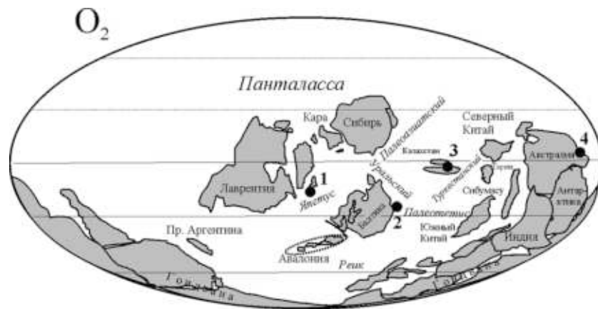
Рис. 43. Местонахождения конодонтов океанической биогеографической области (палеогеография среднего ордовика, по [Scotese, 2001; и др.] с дополнениями) 1 – Южная Шотландия; 2 – Южный Урал; 3 – Казахстан; 4 – Восточная Австралия
