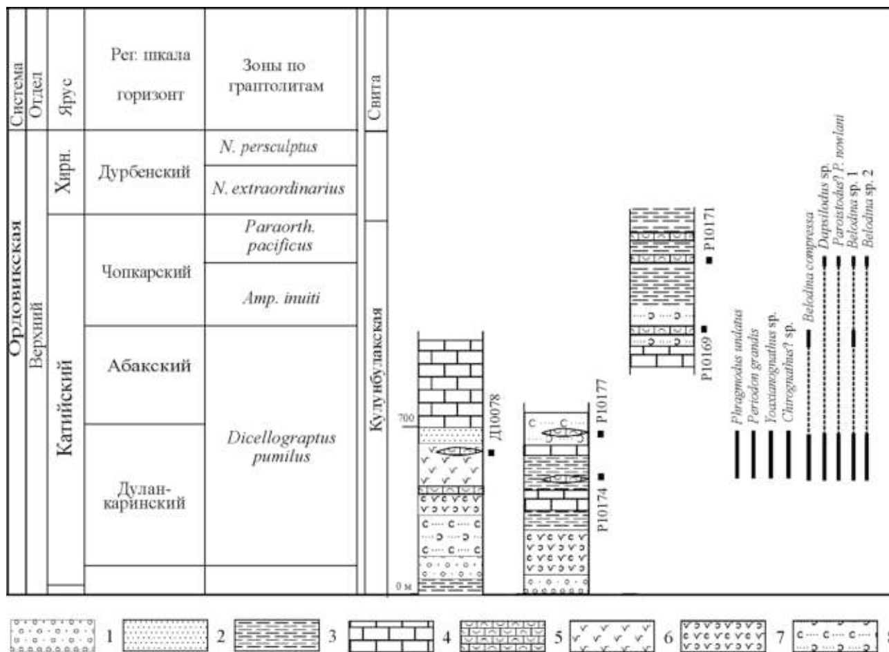
Рис. 27. Разрезы кулунбулакской свиты на правом берегу р. Базар (хр. Тарбагатай) и распространение конодонтов 1 – гравелиты и конгломераты; 2 – песчаники; 3 – алевролиты; 4 – массивные водорослевые известняки; 5 – биокластические известняки; 6 – эффузивы средне-основного состава; 7 – туфы средне-основного состава; 8 – туфопесчаники
