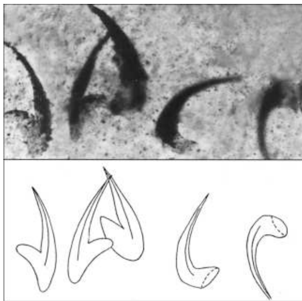
Рис. 68. Группировка из пяти элементов вида Chiganodus parilis в кремнях бурубайтальской свиты, разрез Памятник природы – 9706 (обр. 9 м)
