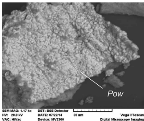
Рис. 2. Снимки с растрового электронного микроскопа выделений повеллита (Pow) и вульфенита (Wul) в пр. 8 рудного интервала Находского U-Mo-Re пункта минерализации
