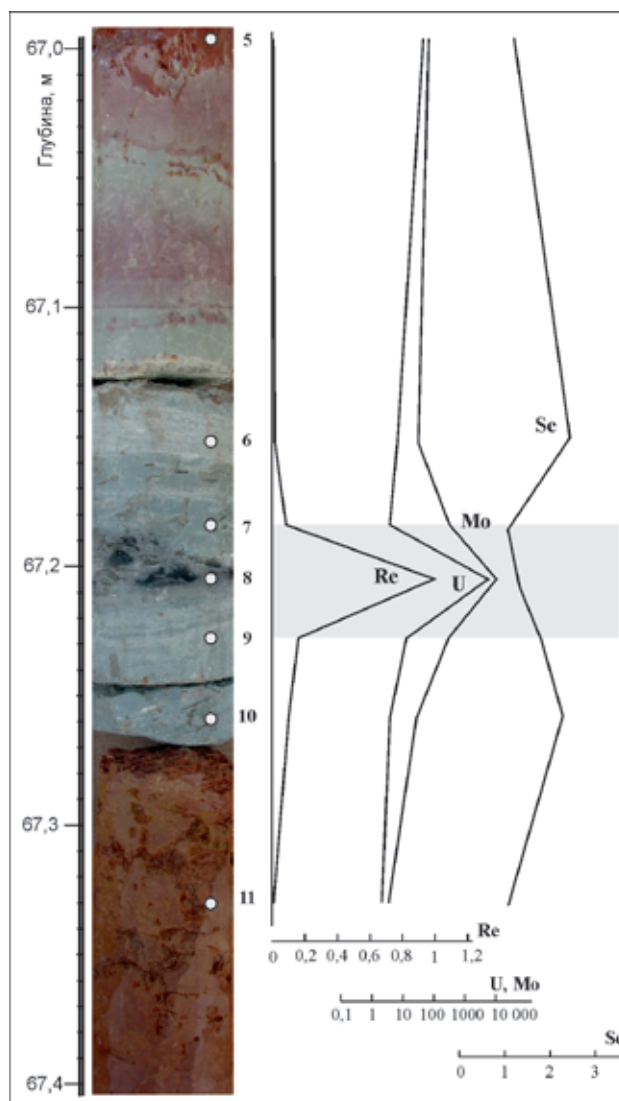
Рис. 1. Разрез скважины Находского пункта U-Mo-Re минерализации с содержанием Re, U, Mo и Se (в г/т)
