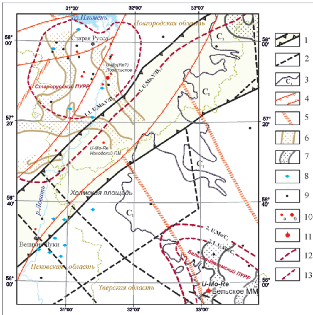
Рис. 3. Схема расположения района исследований относительно близрасположенных потенциальных урановорудных зон, областей и районов
